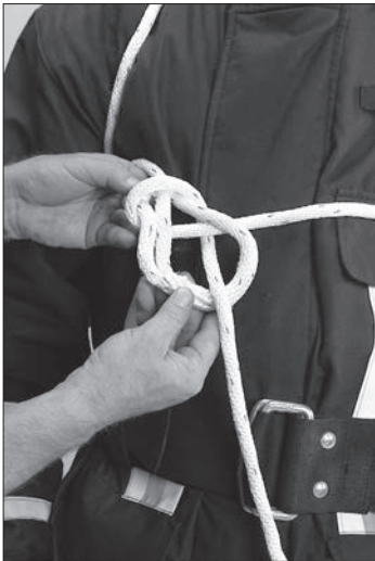
3. Phase – Pfahlstich
